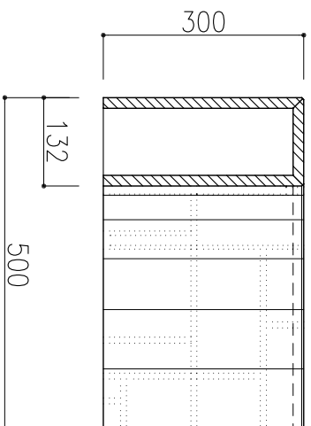
B 立面図 S=1:10
