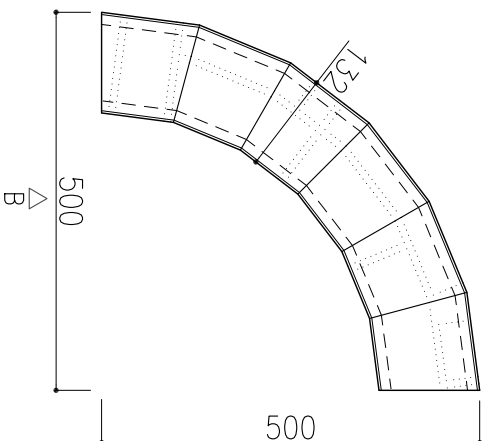
H=300, 400 平面図 S=1:10
