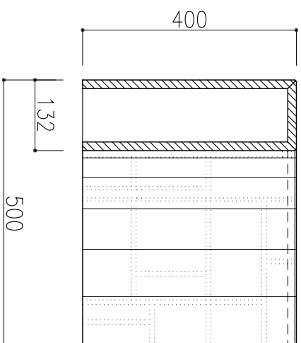
B 立面図 S=1:10
