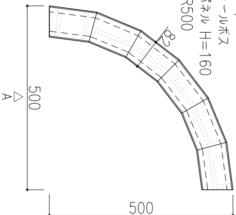
H=160 平面図 S=1:10
